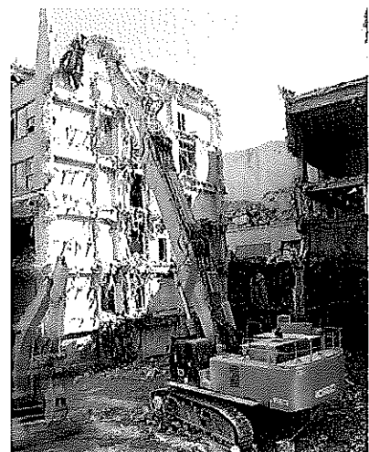
特定解体用機械のコンクリート圧砕機 コベルコ建機株式会社製、同社提供
